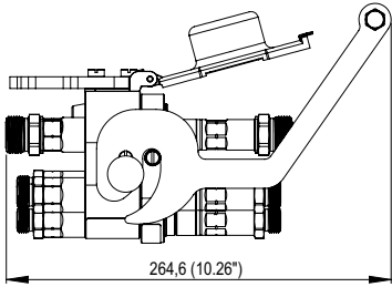
Festhälfte Gekuppelt
