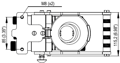
Einbaulage
